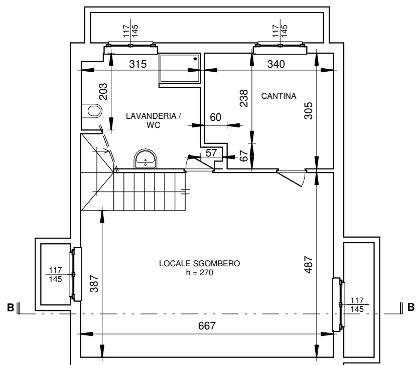
PIANTA PIANO INTERRATO - esistente - sc. 1 : 100
